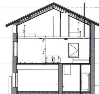
Coupe
